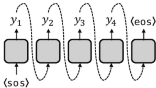
Autoregressive schema
